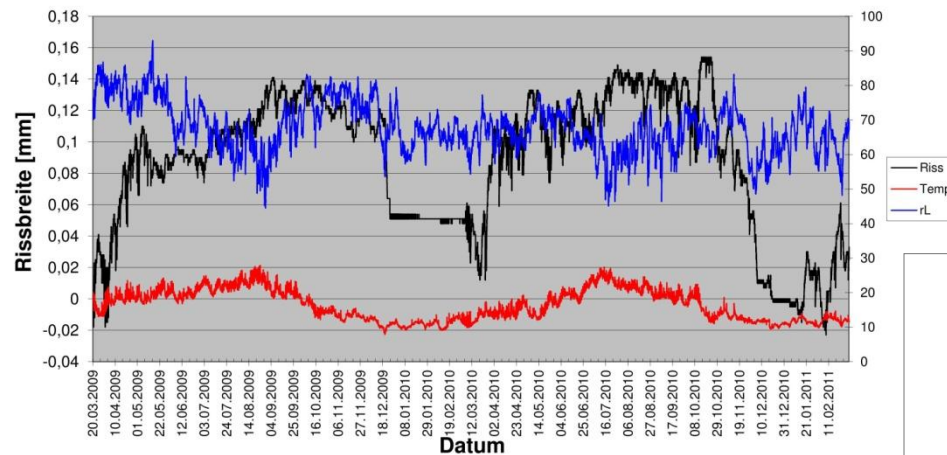
Rissbreite und Klimadaten: Dom, Südseite, unteres Fenster innen
