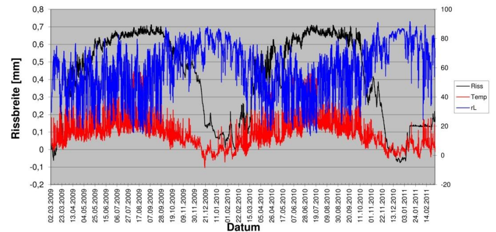
Rissbreite und Klimadaten: Dom, Südseite, außen unten
